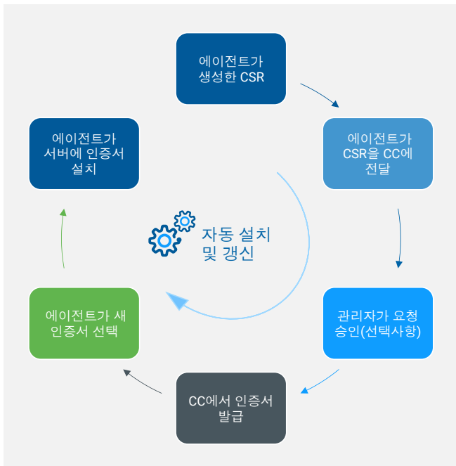
CertCentral® Managed Automation으로 자동화된 인증서 프로비저닝
